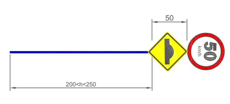
DETALHE 4 - SUPORTE DAS PLACAS EXEMPLO
