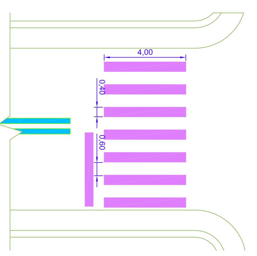
DETALHE 3 - FAIXA DE PEDESTRES
